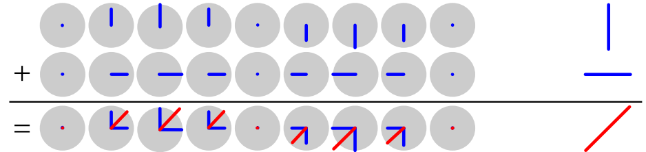
Bild 5: Wellenberge der waagerechten Welle treffen auf einen Wellenberg der horizontalen Welle. Die Addition der Auslenkungen ergibt eine diagonale Welle (rot). Die Auslenkungen liegen also in der diagonalen Ebene, man hat immer noch lineare Polarisation.
